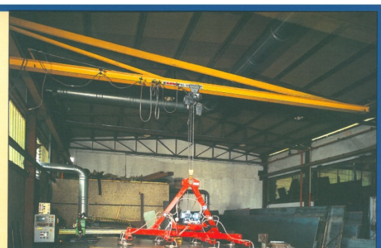
GRU A COLONNA CON VENTOSA TIPO GLA8F Kg. 1000 a 8 piastre rotonde • Column crane with vacuum grab model GLA8F 1000 Kg. with 8 round plates • Grue à colonne avec ventouse type GLA8F 1000 Kg. à 8 plaques rondes • Kran auf Rohrkonstruktion mit Saugnapf des Typs GLA8F aus 8 runden Platten für 1000 Kg. • Grúa de columna con ventosa tipo GLA8F 1000 Kg con 8 planchas redondas.
